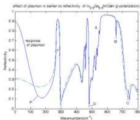
شکل ۸ طیف بازتابی چاه کوانتومی \text{In}_{0.5}\text{Ga}_{0.5}\text{N}/\text{GaN} نالائیده با قطبش P و زاویه تابش 12^\circ .
