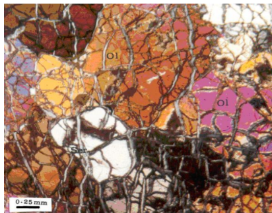
شکل ۲ تصویر میکروسکوپی از قشر دونیتی توده کرومیتی، بلورهای اولیون (Ol) که در حال دگرسانی به سرپانتین هستند. نور PPL.
