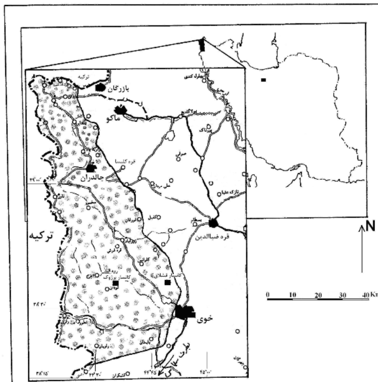
شکل ۱ موقعیت جغرافیایی کانسارهای کرومیت قشلاق و بزروک (مربع‌های توپر) واقع در شمال خاوری خوی. پهنه افیولیتی خوی در شکل نشان داده شده است.
