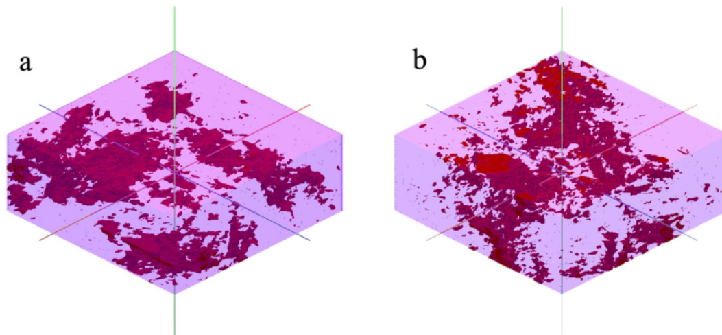
شكل ۸ دو نمونه از مدلهاى فیلتر شده (از مدلهاى a و b شكل ۵) كه نشان دهنده توزيع كانیها در متن سنگ است.
