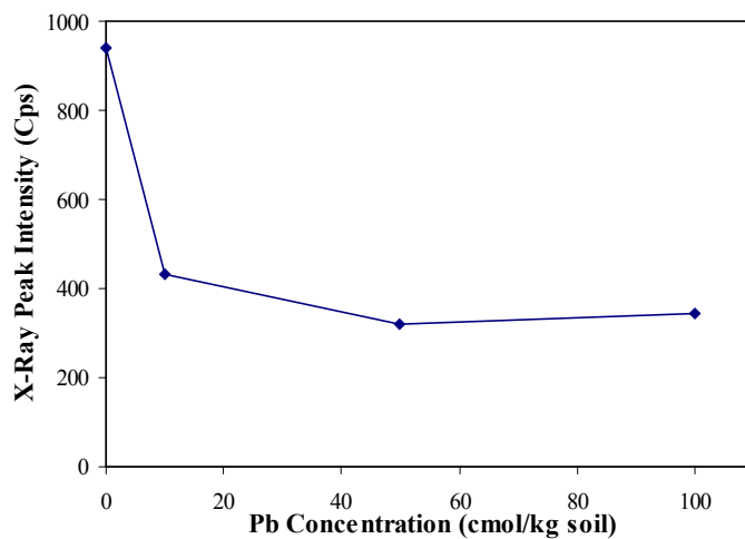
شکل ۹ تغییرات شدت قله اصلی ( 7/1 \text{ \AA} ) در کانی کائولینیت ناشی از افزایش غلظت آلاینده سرب
