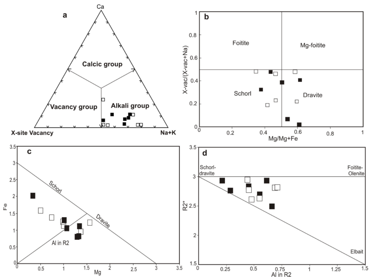
شکل ۳: a: قرار گیری تورمالین‌های منطقه مورد بررسی بر اساس موقعیت X در فرمول تورمالین. b: ترکیب تورمالین در گستره شوریست-دراویت. c: نمودار Fe نسبت به Mg نشانگر قرارگیری نمونه‌ها در زیر خط \sum (Fe+Mg)=3 [۱۶]. d: نمودار R_2^* نسبت به R_2 به
