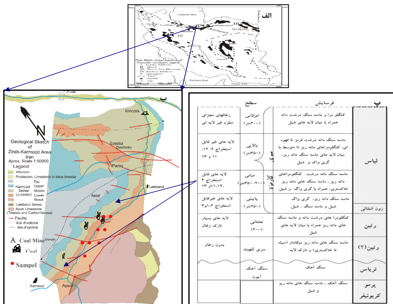
شکل ۱ الف- حوزه‌های اصلی زغال‌سنگ‌های ایران با سن تریاس- ژوراسیک، ب- نقشه زمین‌شناسی منطقه زیرآب- کارمزد، پ- مقطع چین-شناسی منطقه زیرآب - کارمزد (اقتباس از دماگ [۷]).
