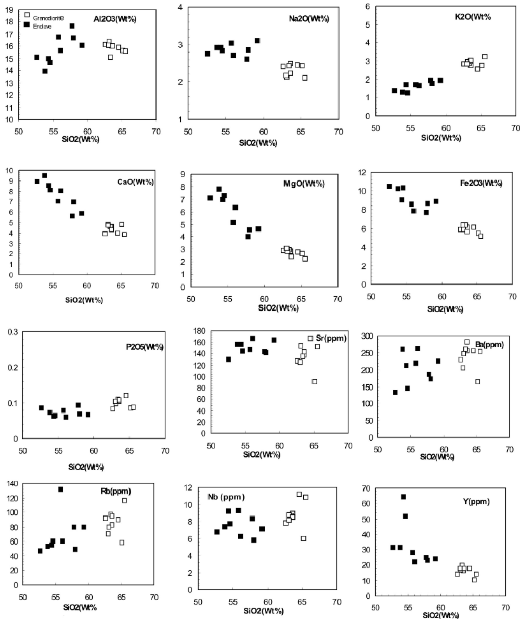
شکل ۵ نمودارهای تغییر عناصر نسبت به میزان SiO 2 [۶]. علائم مشابه شکل ۲ است.
