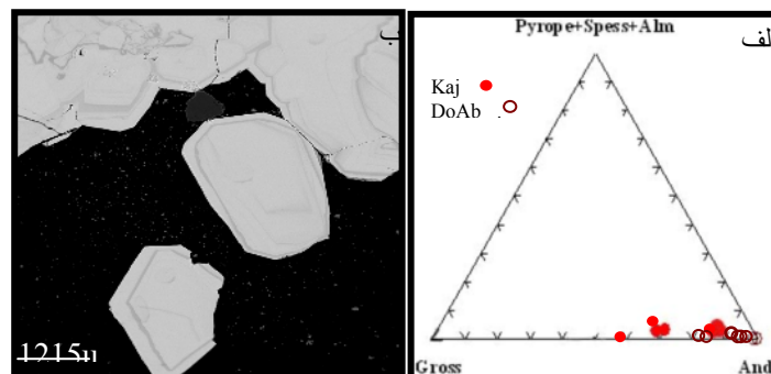
شکل ۱۰ پیدایش گارت‌های آندرادیتی با برجستگی بالا در زمینه‌ای از کلریت (نور عادی).
