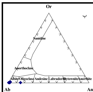
شکل ۹ الف. آلبیت‌های نوظهور در اثر دگرتهادی نمک در سنگ‌های آتشفشانی گنبد نمکی دوآب تشکیل شده است، ب. تشکیل رگچه‌های کوارتز، کلسیت و آلبیت در سنگ‌های آتشفشانی گواه بر تاثیر دگرتهادی در مراحل پایانی تبلور ماگماست (نور قطبیده)، پ. اغلب فلدسپات‌های مورد بررسی روی نمودار تقسیم‌بندی فلدسپات‌ها در گستره آلبیت قرار گرفته‌اند.
