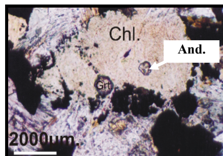
شکل ۱۰ پیدایش گارت‌های آندرادیتی با برجستگی بالا در زمینه‌ای از کلریت (نور عادی).
