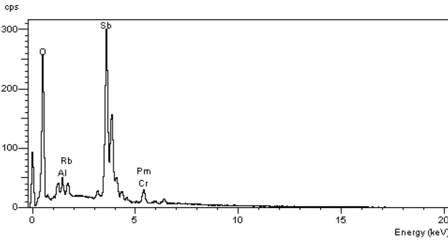
شکل ۹ نمودار آنالیز نقطه‌ای وابسته به نقطه‌ی شماره ۲ در شکل ۷. با میکروسکوپ الکترونی. این ترکیب اکسید آنتیموان حاصل از اکسید شدن استیبنیت در رگه‌های معدنی مورد بررسی است.
