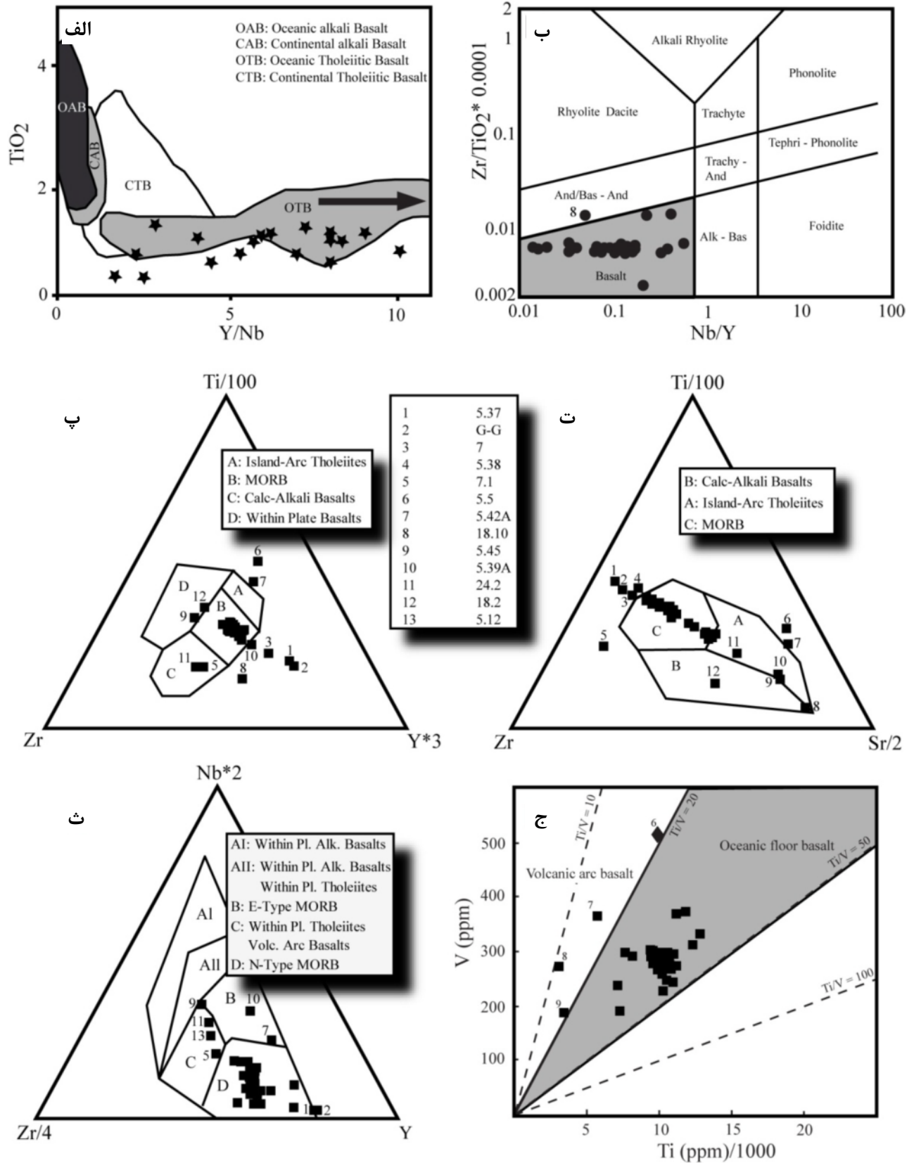
شکل ۴ تقسیم‌بندی شیمیایی سنگ مادر اکلوزیت‌های شاندرمن با استفاده از نمودار (الف) Y/Nb - TiO_2 ، (ب) Zr/TiO_2 - Nb/Y ، (ج) Y/Nb - TiO_2 ، (د) Zr/TiO_2 - Nb/Y ، (ه) Zr/TiO_2 - Nb/Y ، (و) Ti/V نسبت‌ها، پ و ت [۱۸]، ث [۱۹]، ج [۲۰]. (برای اطلاعات بیشتر به متن مقاله مراجعه کنید).
