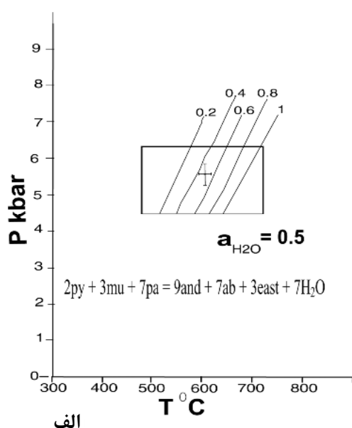
شکل ۵ الف) محاسبه‌ی فعالیت آب در سنگ‌های رسی دگرگون شده گرافیتی بلند پرچین. ب) محاسبه‌ی فعالیت آب در سنگ‌های رسی دگرگون شده غیرگرافیتی پشتوک. علائم اختصاری کانی‌ها عبارتند از کوآرتز= q، مسکویت= mu، پاراگونیٹ= pa، آلبیت= ab، استونیت= east، کلریتوئید= ctd، آلماندین= alm، استارولیت آهن دار= fst.
