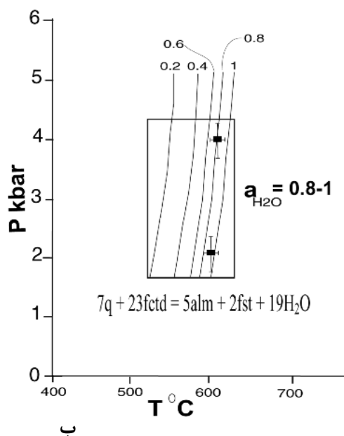
شکل ۵ الف) محاسبه‌ی فعالیت آب در سنگ‌های رسی دگرگون شده گرافیتی بلند پرچین. ب) محاسبه‌ی فعالیت آب در سنگ‌های رسی دگرگون شده غیرگرافیتی پشتوک. علائم اختصاری کانی‌ها عبارتند از کوآرتز= q، مسکویت= mu، پاراگونیٹ= pa، آلبیت= ab، استونیت= east، کلریتوئید= ctd، آلماندین= alm، استارولیت آهن دار= fst.
