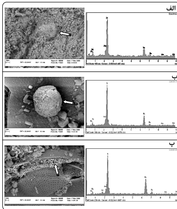
شکل ۳ تصاویر میکروسکوپ الکترونی و آنالیز EDS پیریت در رسوب‌های دریایی گودال نانکای. الف) تشکیل پیریت فرمبوتیدال در زمینه رسوب‌ها. ب و پ) تشکیل پیریت اتوژنیک و فرمبوتیدال در حجره فرمینفرا.
