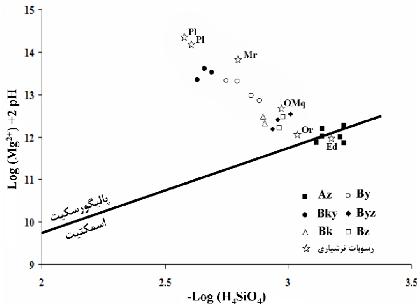
شکل ۸ نمودار پایداری سیستم پالیگورسکیت-اسمکتیت بر اساس ترکیب شیمیایی نمونه‌های خاک و مواد مادری مورد بررسی که بیانگر پایداری بیشتر پالیگورسکیت در افق‌های انباشت گچ نسبت به افق‌های انباشت آهک و نمک، و ناپایداری نسبی این کانی در برخی افق‌های سطحی و رسوب‌های ائوسن است.
