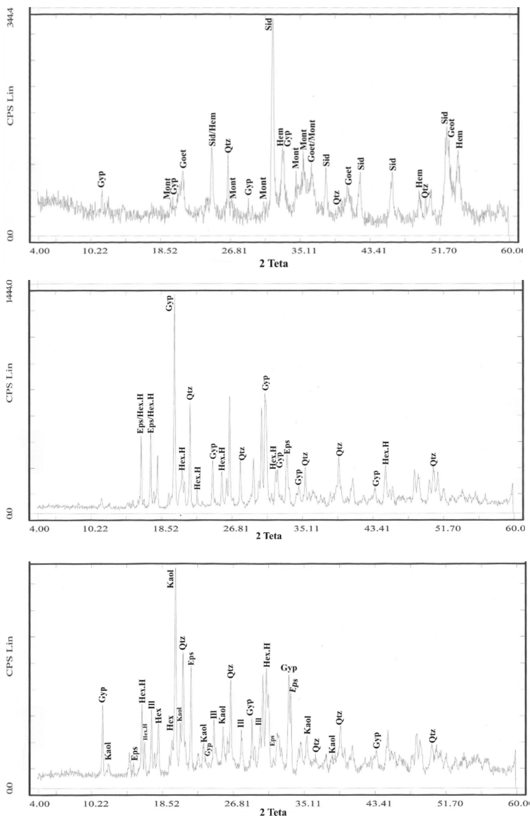
شکل ۵ سه نمونه از الگوی‌های پراش پرتو ایکس (XRD) کانی‌های ثانویه (زیست محیطی) تشکیل شده در سطوح انبارهای باطله‌ی جدید کارخانه زغال‌شویی وطنی (ژپس=Gyp، مونت موریلونیت=Mont، گوتیت=Goet، سیدریت=Sid، همتایت=Hem، کوارتز=Qtz، اپسومیت=Eps، هگزا هدریت=Hex.H، کائولینیت=Kaol، ایلیت=Ill).
