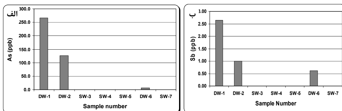
شکل ۴ الف) مقدار آرسنیک در نمونه‌های آب منطقه‌ی معدنی چشمه زرد و ب) مقدار آنتیموان در نمونه‌های آب منطقه‌ی معدنی چشمه زرد (آب آشامیدنی DW و آب چشمه‌ی SW نامگذاری شده است).
