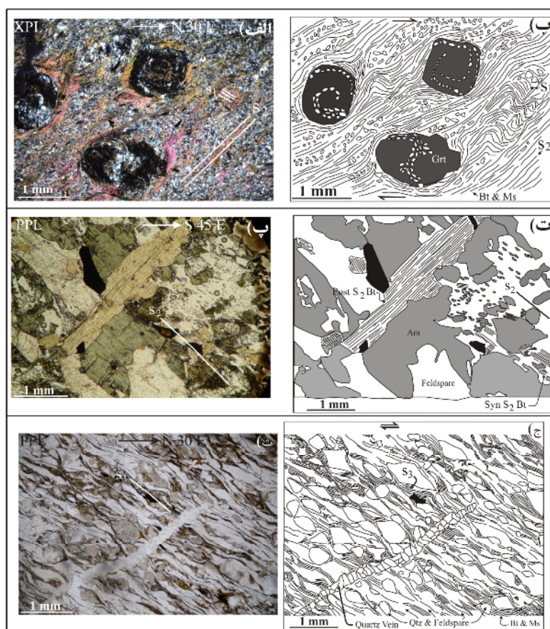
شکل ۵ الف، ب: چند ترکیبی‌های گارنت‌ها در فیلیت‌ها و شیست‌های رسوبی همبافت روتشون که همزمان با شیستوزیته S_2 تشکیل شده‌اند؛ پ، ت: پورفایروبلست‌های بیوتیت در سنگ‌های بازی همبافت گل‌گهر که روی شیستوزیته S_2 رشد کرده‌اند؛ ث، ج: فاز دگرشکلی D_3 باعث تبدیل شدن سنگ به میلونیت و ایجاد شیستوزیته محلی S_3 شده است. در این نمونه بلورهای کوارتز و فلدسپات به صورت عدسی‌هایی کشیده دیده می‌شوند که از طرفین به وسیله ریزبلورهای موسکویت و بیوتیت و از دو انتها نیز با ریزبلورهای کوارتز احاطه شده‌اند.
