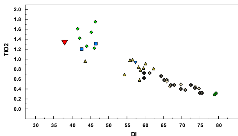
شکل ۲۹ نمودار تغییرات TiO_2 نسبت به شاخص تفريق.
