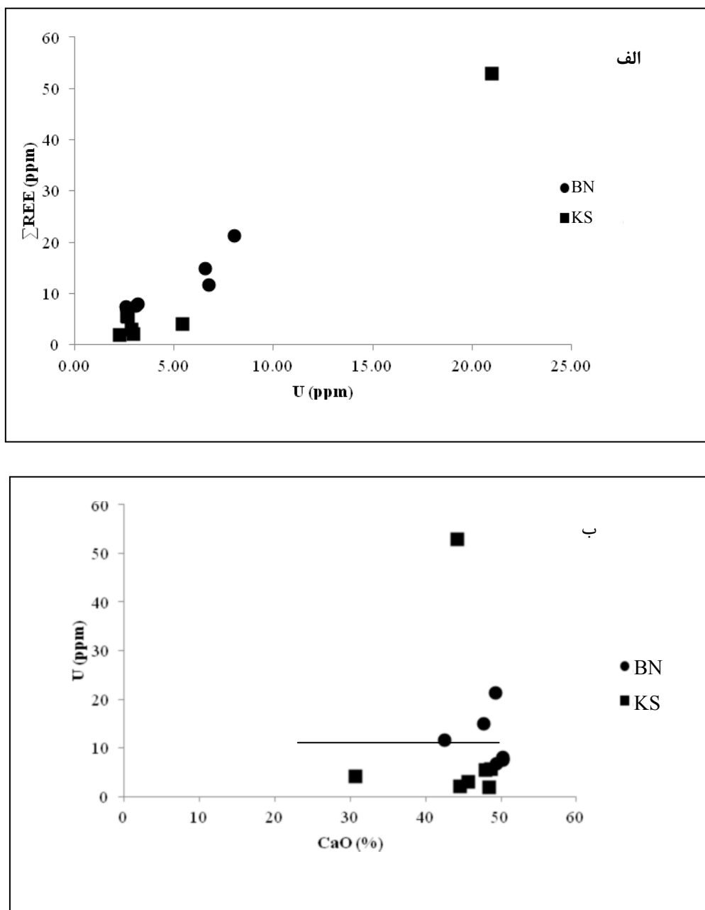
شکل ۴ الف- ارتباط مستقیم بین تغییرات U و \Sigma\text{REE} نشان دهنده‌ی این است که اورانیوم و REE ها خاستگاه مشترکی در فسفریت‌ها دارند ب- رابطه‌ی معکوس بین U و CaO منعکس کننده‌ی عدم ارتباط بین آنها است
