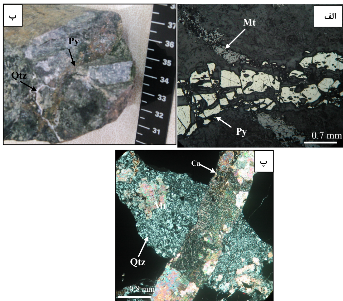
شکل ۱۱ الف) تصویر میکروسکوپی از رگچه سولفیدی نسل سوم (Py) که رگه مگنتیتی را قطع کرده است، (PPL؛ ب) تصویر نمونه‌ی دستی از رگه‌ی سیلیسی تأخیری (Qtz) که رگه‌ی سولفیدی (Py) را قطع کرده است، پ) تصویر میکروسکوپی از رگچه کربناتی (Ca) تأخیری که رگچه سیلیسی تأخیری (Qtz) را قطع کرده است (XPL).
