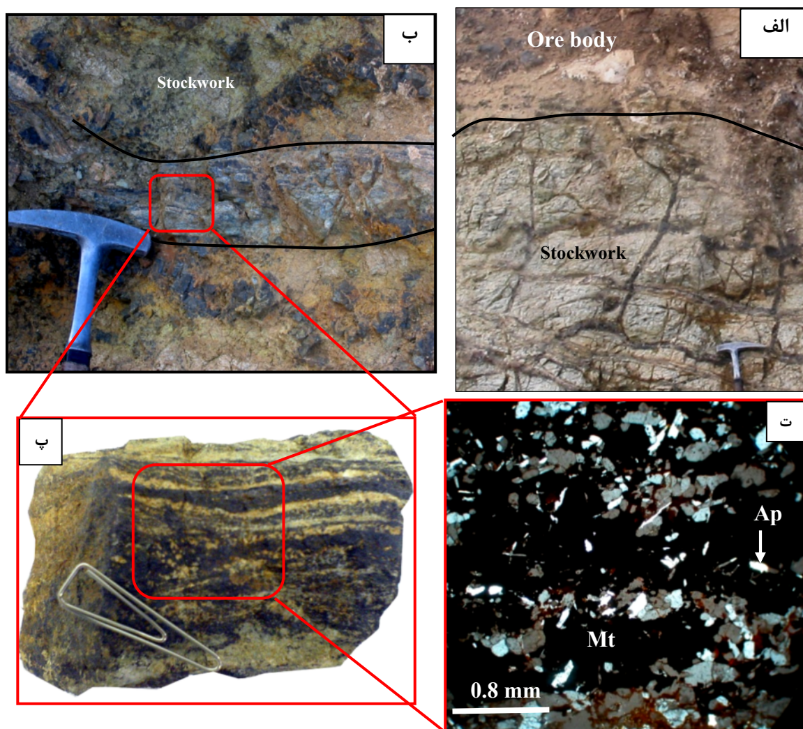
شکل ۵ الف) ساخت و بافت داربستی در بخش زیرین ماده‌ی معدنی و در درون توده‌ی نفوذی به شدت دگرسان شده، ب) تصویر نزدیک‌تر از رگه‌های داربستی، که دارای بافت نواری بین مگنتیت و آپاتیت است، پ) نمونه‌ی دستی از رگه داربستی دارای بافت نواری در تصویر (ب، ت) تصویر میکروسکوپی از نمونه‌ی دستی بخشی از تصویر (پ)، که حامل نوارهای غنی از آپاتیت (Ap) در مگنتیت (Mt) است (XPL).
