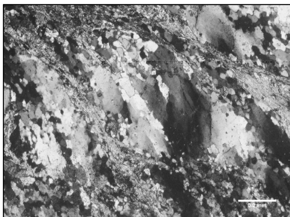
شکل ۸ ریزساختار هسته و گوشته در بلورهای کوارتز در میلونیت‌های هسته‌ی گسل‌های مورد بررسی. این ساختار مراحل ابتدایی اقلیم باز تبلور دینامیکی SGR را نشان می‌دهد.
