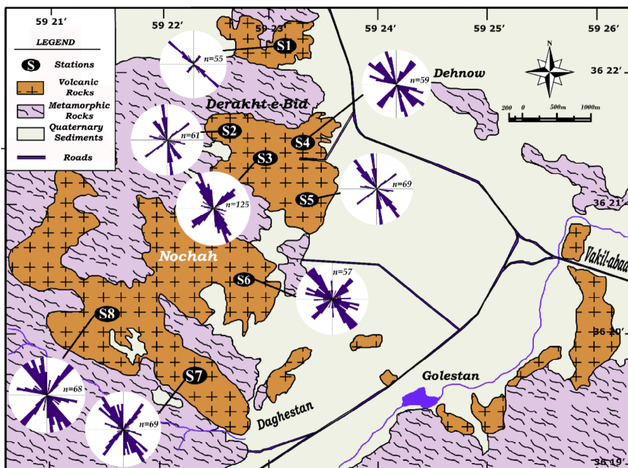
شکل ۲ نقشه‌ی زمین‌شناسی گستره‌ی مورد بررسی. نمودارهای گل‌سرخ سمت‌گیری رده‌های شکستگی‌های منظم در توده‌ی تونالیتی درخت بید را نشان می‌دهند.
