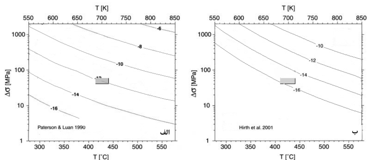
شکل ۱۲ نمودار تنش تفاضلی- دما و نرخ کرنش در میلونیت‌ها (اقتباس از [۲۰]). منحنی‌ها در نمودار نرخ کرنش را نشان می‌دهند. نمودار (الف) بر پایه‌ی مدل ارائه شده توسط [۳۰] و نمودار (ب) بر پایه مدل ارائه شده توسط [۳۱] ترسیم شده‌اند. چهار گوشه‌ها گستره‌ی نرخ کرنش را در میلونیت‌های مورد بررسی در دو مدل [۳۰، ۳۱] نشان می‌دهند.
