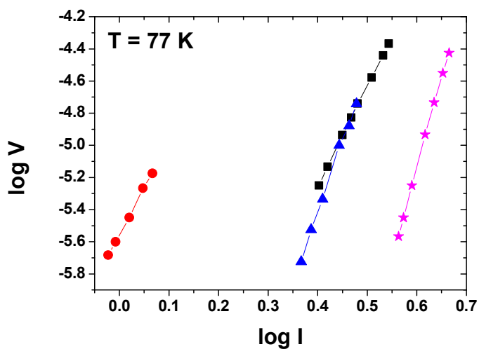
شکل ۸ نمودار \log V - \log I برای نمونه‌های آلیش شده با مقادیر مختلف نانوذرات طلا (●) ۰٫۵٪، (▲) ۱٪ و (★) ۲٪ با زمان پخت ۷۲ ساعت.
