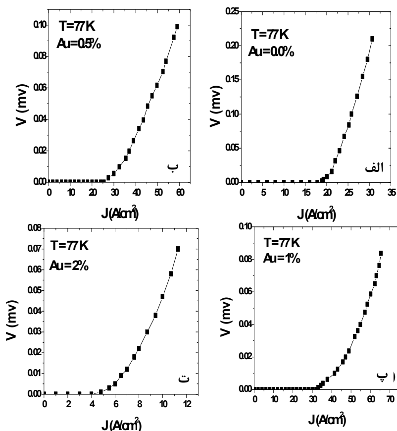
شکل ۵ نمودارهای V-J برای مقادیر متفاوت نانوذرات طلا (الف، ۰٫۵٪، ب، ۰٫۵٪، پ) و ۲٪ (ت) با زمان پخت ۷۲ ساعت.
