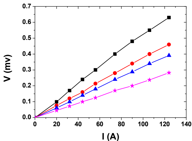
شکل ۶ نمودار V-I برای نمونه‌های آلیش داده شده در دمای اتاق با مقادیر مختلف نانوذرات طلا (■) ۰٫۵٪، (●) ۰٫۵٪، (▲) ۱٪ و (★) ۲٪ با زمان پخت ۷۲ ساعت.
