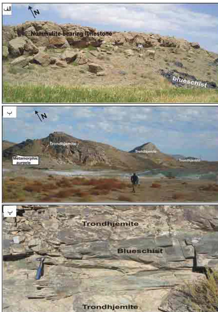
غشکل ۲ الف- رسوب‌گذاری آهک‌های نومولیت‌دار به‌صورت دگرشیب روی شیست‌های آبی جنوب‌غربی خوشاب. ب- تزریق سیل مانند توده‌های ترونجمیتی به درون مجموعه‌ی دگرگونی که با تشکیل هاله‌ی دگرگونی محدود نیز همراه است. پ- زنولیت شیست آبی که به وسیله‌ی توده‌ی ترونجمیتی در بر گرفته شده است.
