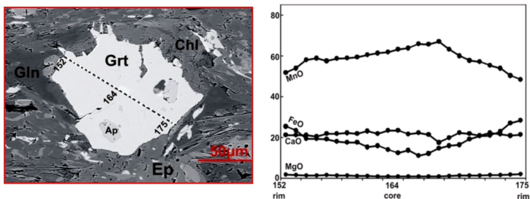
شکل ۷ تصویر BSE گارنت و الگوهای منطقه‌بندی آن در انواع نسل اول شامل کاهش Mn و افزایش \text{Fe}^{2+} و Mg از مرکز به حاشیه‌ی بلور است و بیانگر رشد گارنت در مرحله‌ی دگرگونی پیش‌رونده است. افزایش Mn، نسبت \text{Fe}^{2+}/\text{Mg} و کاهش Fe در خارجی‌ترین بخش گارنت نیز موید تبادلات یونی طی دگرگونی پس‌رونده است.
