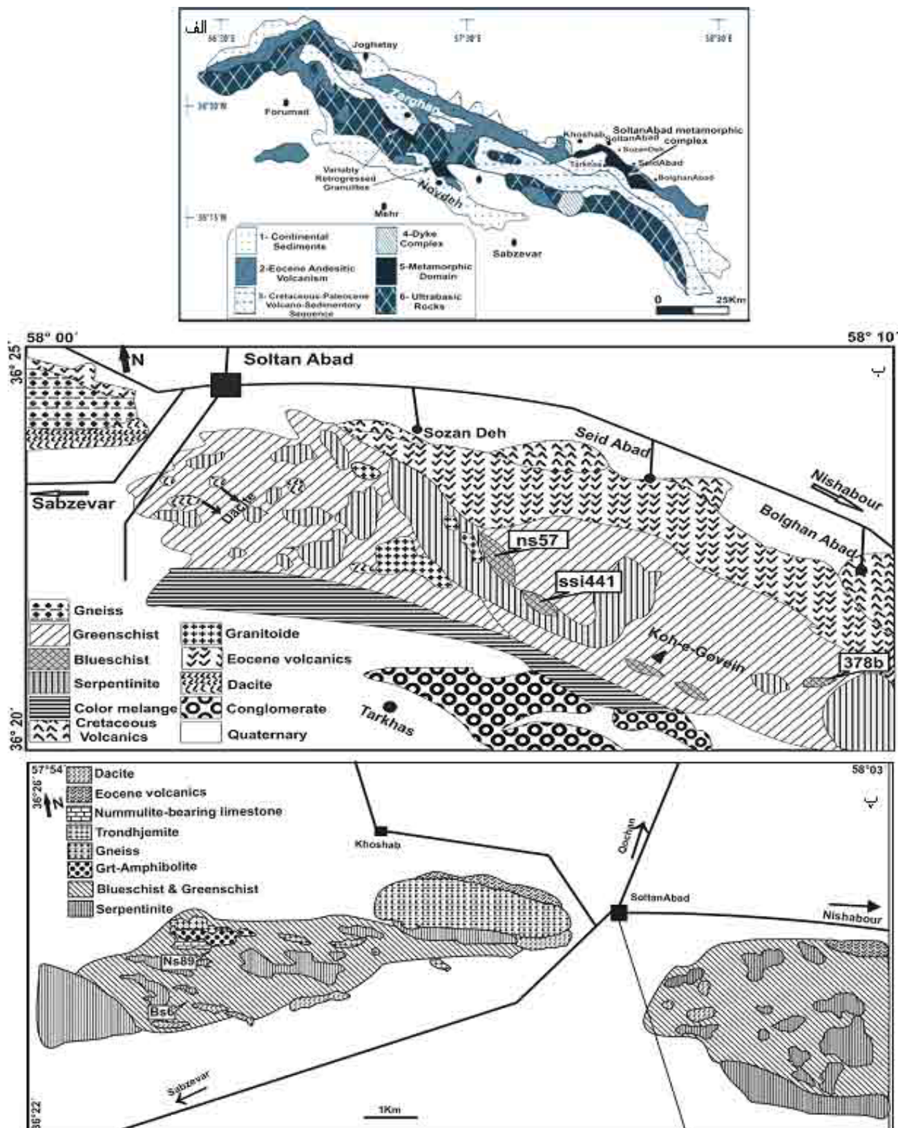
شکل ۱- الف- نقشه‌ی زمین‌شناسی ساده شده از نوار افیولیتی شمال سبزوار و مجموعه‌ی دگرگونی سلطان‌آباد که در شمال‌شرقی سبزوار قرار دارد (با تغییرات از [۱۸]). ب- نقشه‌ی زمین‌شناسی ساده شده از نوار دگرگونی جنوب‌شرقی سلطان‌آباد (با تغییرات از [۱۹]). پ- نقشه‌ی زمین‌شناسی ساده شده از نوار دگرگونی غرب و جنوب‌غربی سلطان‌آباد. محل نمونه‌برداری شیست‌های آبی روی این نقشه‌ها مشخص شده است.
