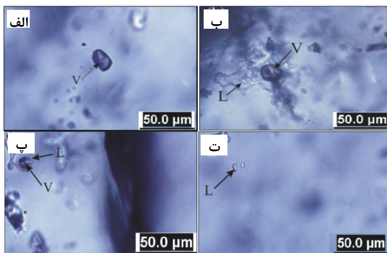
شکل ۸ الف) شاره‌ی درگیر تک فاز گاز (V)، ب) شاره‌ی درگیر دو فاز (L) فاز مایع و (V) فاز گاز، پ) شاره‌ی درگیر تک فاز آبیگن (L)، ت) شاره‌ی درگیر دو فاز (V) فاز گاز و (L) فاز آبیگن.
