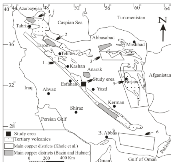
شکل ۱ مناطق اصلی کانسار سازی مس در ایران: (۱) کمربند ارومیه- دختر (۲) ناحیه البرز غربی (۳) ناحیه کویر- سبزوار (۴) ناحیه سبلان (۵) ناحیه لوت (۶) ناحیه مکران، برگرفته از [۱۷].
