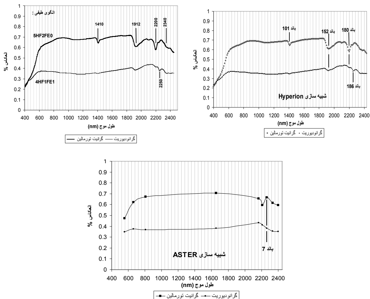
شکل ۱۱ مقایسه طیف آزمایشگاهی با شبیه سازی همان طیف‌ها بر اساس دو سنجنده فراطیفی و چند طیفی.
