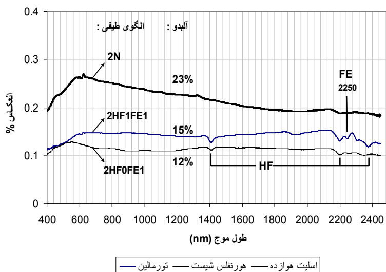
شکل ۸. مقایسه طیف‌ها با توجه به الگوهای جذب، الگوی طیفی، کلاس آلدو و شدت جذب.
