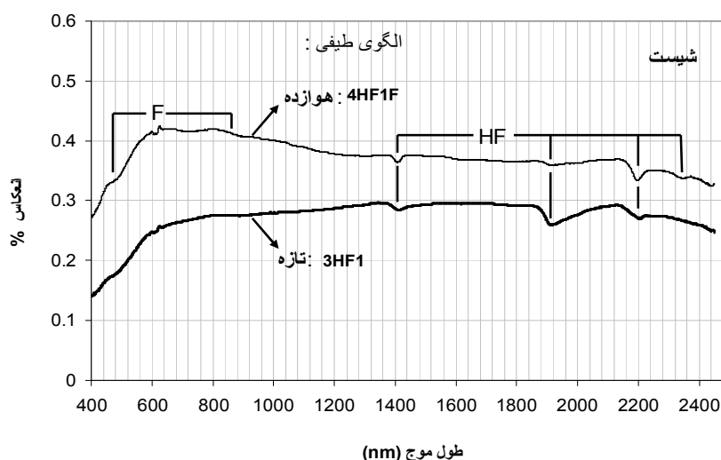
شکل ۹ مقایسه الگوهای جذب، الگوهای طیفی و میزان آلودگی کلی در طیف های دو سنگ شیتست تازه و هوازده.
