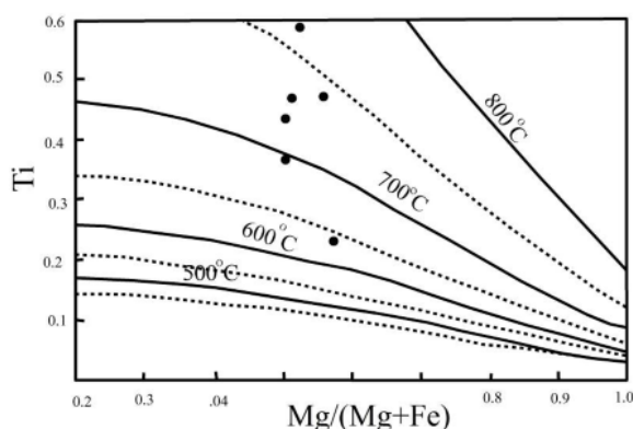
شکل ۸. نمودار همدمای زمین دماسنج تیتانیوم در بیوتیت [۱۷].
