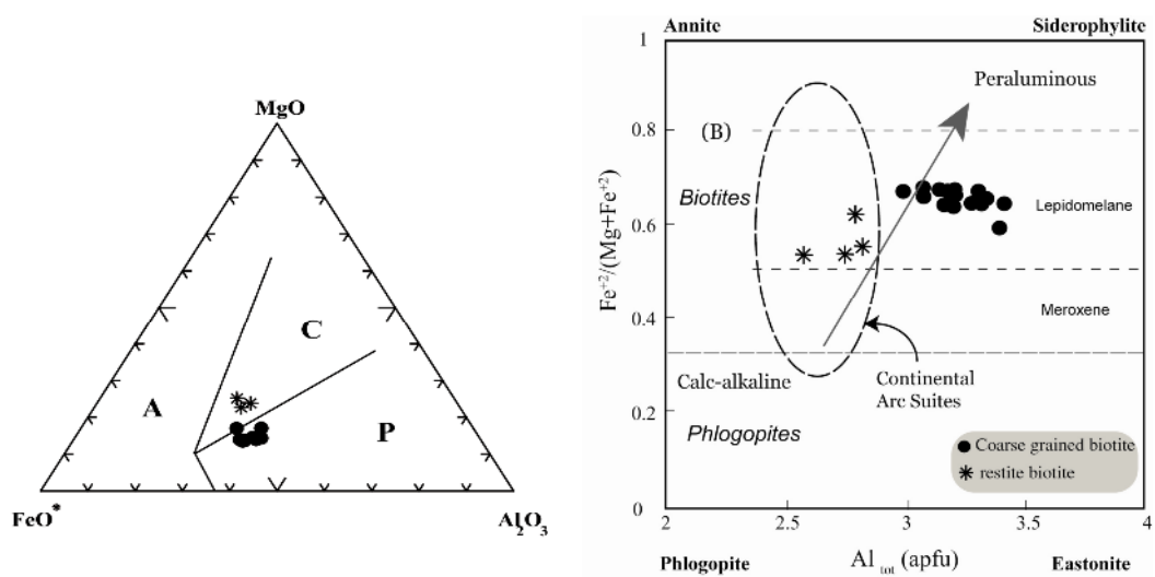
شکل ۲ الف) رده‌بندی میکاها با استفاده از ترکیب شیمیایی آن‌ها [۸]. ب) نمودار مثلثی اکسیدهای MgO, Al 2 O 3 و FeO* [۹] برای تعیین محیط زمین‌ساختی گرانیت‌ها با استفاده از اکسیدهای MgO, Al 2 O 3 و FeO* موجود در ساختار بیوتیت. A: بیوتیت در جایگاه‌های آلکان غیر کوهزایی؛ P: بیوتیت در جایگاه‌های پرآلمین (شامل گرانیت‌های نوع S)؛ C: بیوتیت در جایگاه‌های آهکی-قلیایی کوهزا.
