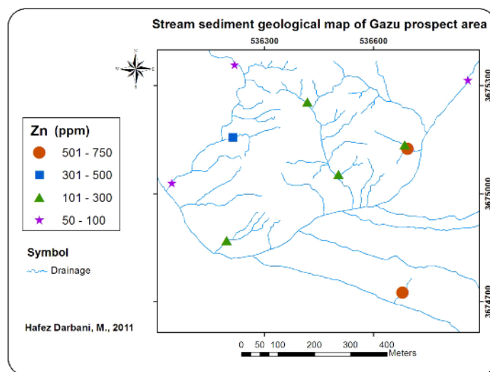
شکل ۱۳ پ نقشه‌ی ژئوشیمی رسوب‌های آبراهه‌های عنصر روی، گستره‌ی پی‌جویی گزو.
