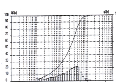
شکل (۵-الف). تعیین گستره‌ی قطر ذرات نمونه بنتونیت
