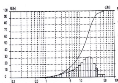
شکل (۵-ب). تعیین گستره‌ی قطر ذرات نمونه‌ی نانورس صنعتی کلوزایت \text{Na}^+
