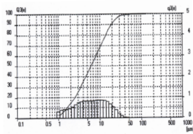
شکل (۵-پ). تعیین گستره‌ی قطر ذرات نمونه نانو رس آزمایشگاهی SLB
