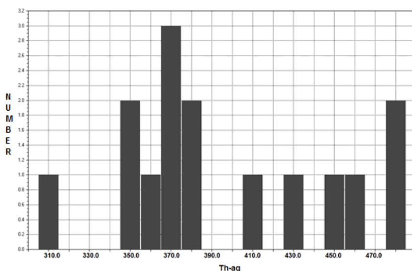
شکل ۱۳ نمودار ستونی دمای همگن شدن نسبت به فراوانی میانبرهای شاری نمونه‌های مورد بررسی.
