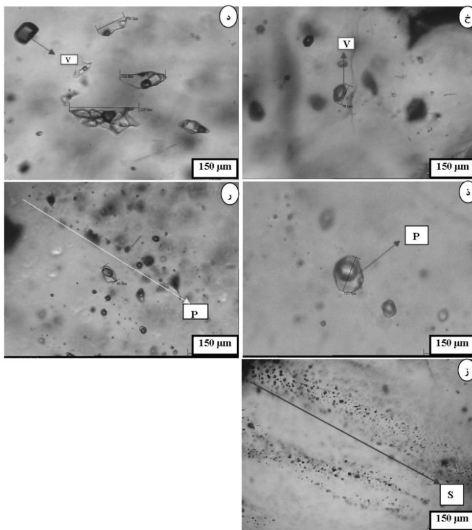
شکل ۹ خ، د، میانبرهای شاری تک فاز گاز د، میانبرهای شاری اولیه ر، تصاویر میانبرهای شاری ثانویه ی کاذب ز، تصاویر میانبرهای شاری ثانویه.
