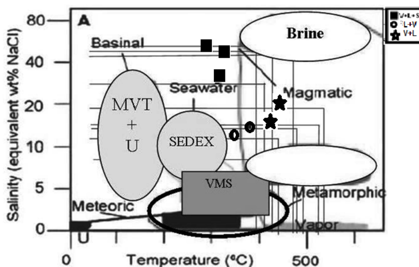
شکل ۱۴ نمودار دمای هموزن شدن نسبت به درجه‌ی شوری میانبرهای شاری نمونه‌های بررسی شده که انواع B, C دارای خاستگاه ماگمایی بوده ولی نوع A خاستگاه جوی و شورابها دارد [۲۲].
