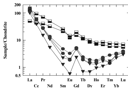
شکل ۶ عناصر نادر خاکی بهنجار شده به کندریت بر اساس [۲۱].
