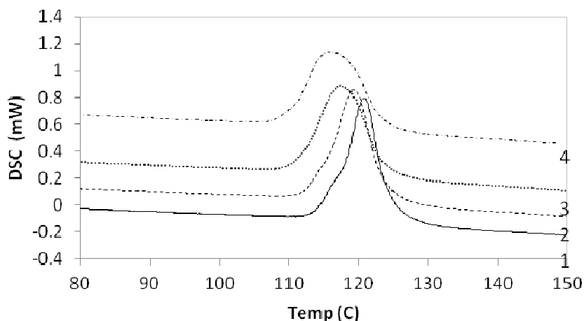
شکل ۷ منحنی DSC پلی پروپیلین سرد شده در (۱): هوا، (۲) کاست، (۳): تحت فشار و (۴): ازلت.
