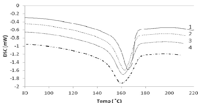
شکل ۶ منحنی DSC پلی پروپیلین ذوب شده در (۱): هوا، (۲) کاست، (۳): تحت فشار و (۴): ازلت.
