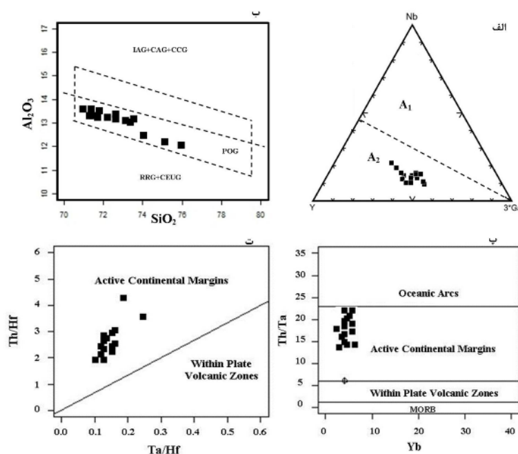
شکل ۹ (الف) در نمودار سه تایی Y-Nb-3×Ga، نمونه‌ها در قلمرو A 2 قرار می‌گیرند [۳۹، ۲۵]، (ب) در نمودار Al 2 O 3 نسبت به SiO 2 [۵۵] نمونه‌ها در گستره‌ی بسا از کوهزائی قرار می‌گیرند، پ و ت) در نمودار تعیین محیط زمین‌ساختی نمونه‌ها در گستره‌ی حاشیه قاره‌ای قرار می‌گیرند [۵۶].
