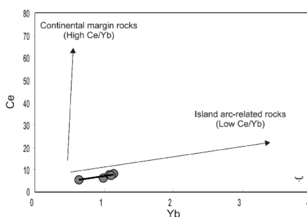
شکل ۹ الف) نمودار La/Yb نسبت La نشان می‌دهد که تحول ماگما بیشتر تحت تاثیر ذوب بخشی است. ب) تغییرات میزان Yb نسبت به Ce برای سنگ‌های گابرویی مورد بررسی. روندهای جزایر قوسی ( Ce/Yb پایین) و حاشیه‌ی قاره‌ای ( Ce/Yb بالا) از [۲۶].
