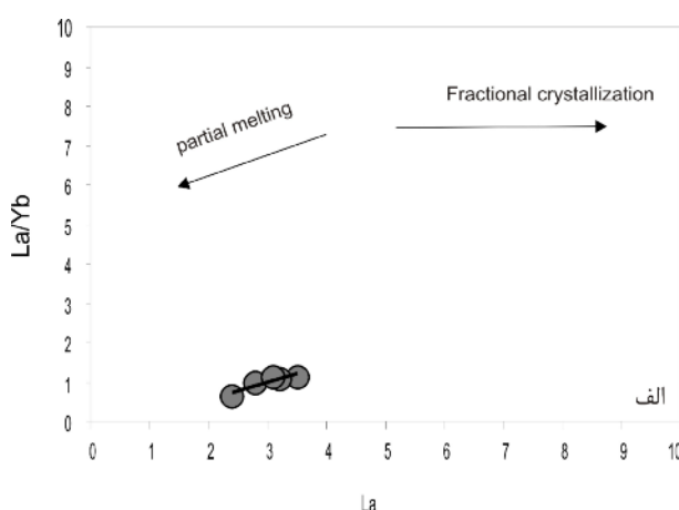
شکل ۹ الف) نمودار La/Yb نسبت La نشان می‌دهد که تحول ماگما بیشتر تحت تاثیر ذوب بخشی است. ب) تغییرات میزان Yb نسبت به Ce برای سنگ‌های گابرویی مورد بررسی. روندهای جزایر قوسی ( Ce/Yb پایین) و حاشیه‌ی قاره‌ای ( Ce/Yb بالا) از [۲۶].
