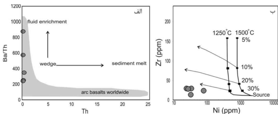
شکل ۱۲ الف) نمودار Ba/Th بر حسب Th نشاندهنده‌ی نقش شاره‌های آزاد شده از پوسته‌ی فرورونده در تشکیل ماگمای گابروهای مورد بررسی است [۵۲] ب) نمودار Zr/Ni بر حسب Ni برای سنگ‌های مورد بررسی (برگرفته از [۵۰]).
