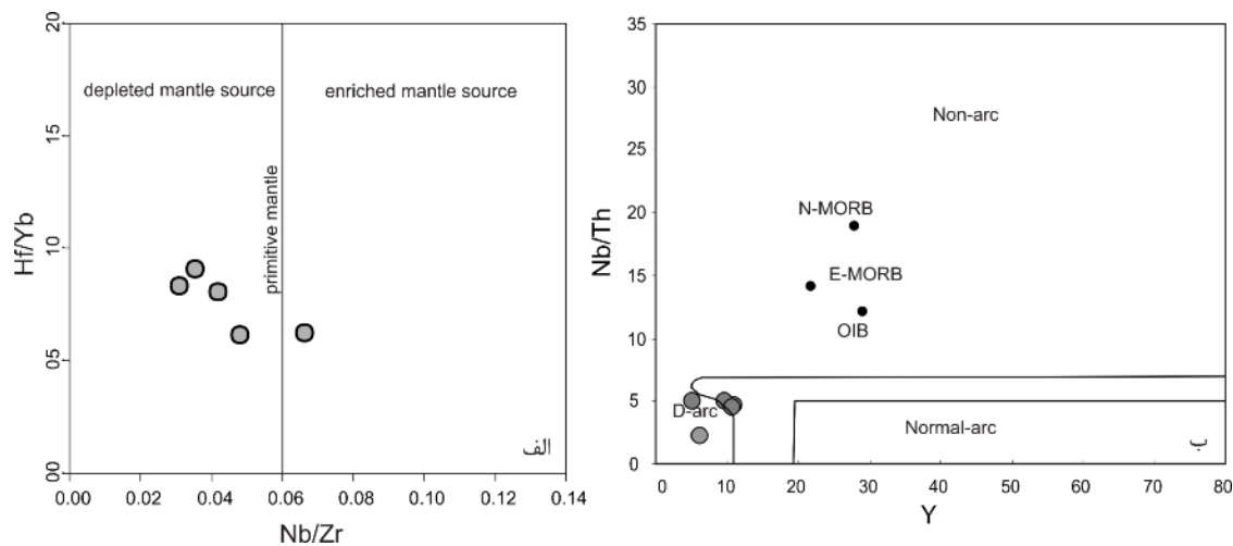
شکل ۱۳ الف) در نمودار Hf/Yb نسبت به Nb/Zr (با تغییرات از [۵۳]) گابروها در بخش دارای مقادیر پایین Nb/Zr قرار می‌گیرند. ب) نمودار D-arc Nb/Th-Y: کمان تهی‌شده. ترکیبات نمایشی بازالت اقیانوسی غیرکمان از [۲۵] است. نمونه‌های مورد بررسی در گستره‌ی کمان قرار می‌گیرند.
