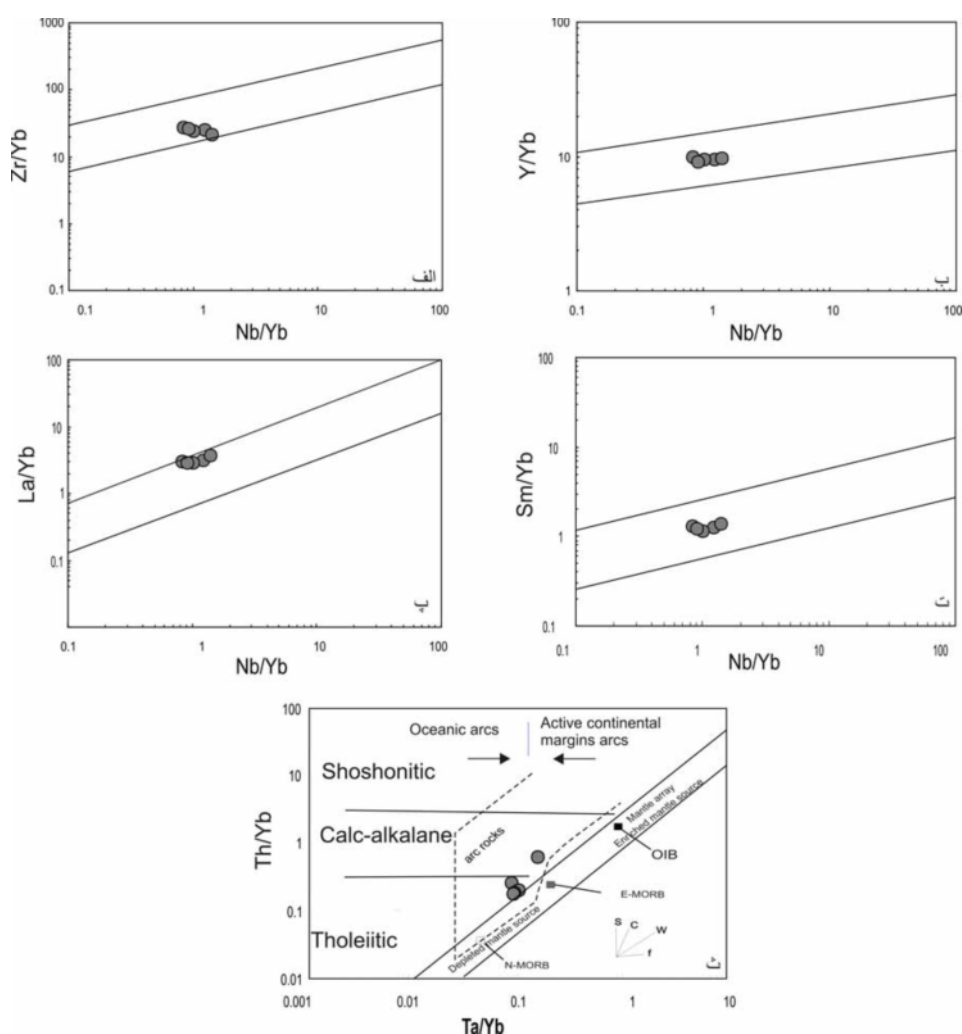
شکل ۱۱ نمودار M/Yb نسبت به Nb/Yb سنگ‌های گابرویی بغم. الف) Zr/Yb ب) Y/Yb پ) La/Yb و ت) Sm/Yb MORB و OIB به ترتیب معرف خاستگاه گوشته جزایر اقیانوسی و پشتی میان اقیانوسی است. آرایه گوشته‌ای (آرایه OIB-MORB) اقتباس از [۵۱]. ث) نمودار Th/Yb بر حسب Ta/Yb با آرایه‌ی گوشته‌ای اقتباس از Pearce (1983) که s نشان‌دهنده‌ی نقش اجزای درگیر در فرورانش، c آلودگی پوسته‌ای، w غنی‌شدگی درون صفحه‌ای و f تبلور بخشی.
