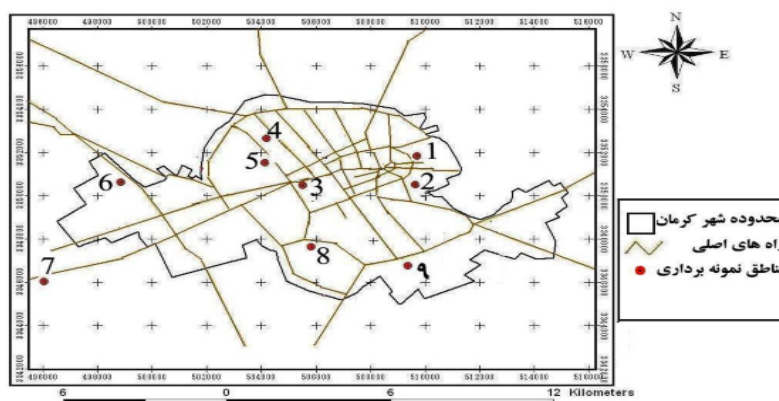
شکل ۴ موقعیت نقاط نمونه برداری غبار در شهر کرمان: (محدوده‌ی زیرسیف (۱)، مدیریت (۲)، میدان آزادی (۳)، شهرک شهید باهنر (۴)، انتهای بلوار شیراز (۵)، شهرک هوانیروز (۶)، شهرک صنعتی (۷)، میدان ابودر (۸)، دانشگاه شهید باهنر (۹)).
