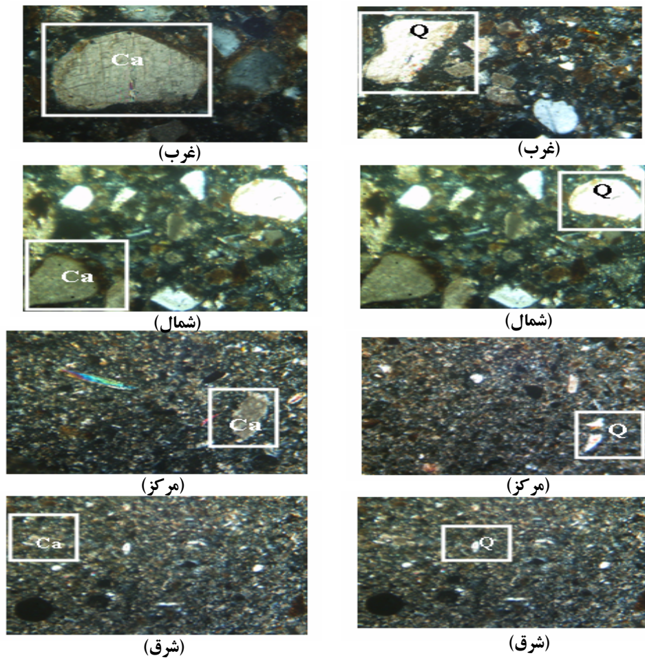
شکل ۱۳ روند تغییر در اندازه های کانی های کلسیت و کوارتز در غبار مناطق مختلف شهر کرمان.
