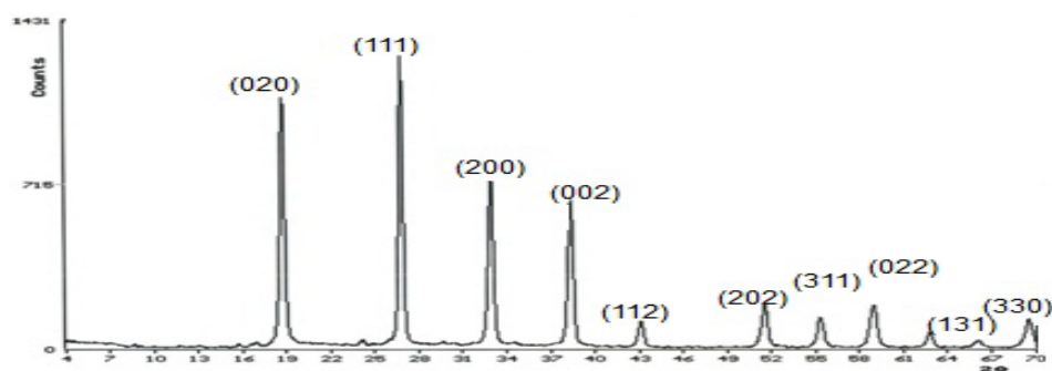
شکل ۳ الگوی XRD متاسیلیکات لیتیم با نسبت مولی ۱:۲ Li:Si در شرایط دمایی 180^{\circ}\text{C} و طول زمان ۷۲ ساعت به روش گرمایی.
