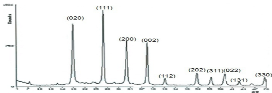
شکل ۱ الگوی XRD متاسیلیکات لیتیم با نسبت مولی ۱:۱ Li:Si در شرایط دمایی 180^{\circ}\text{C} و مدت زمان ۷۲ ساعت به روش گرمایی.
