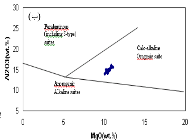
شکل ۹ الف و ب ترسیم اکسیدهای Al_2O_3 و FeO ، MgO بیوتیت‌های مورد بررسی در نمودارهای [۲۴].
