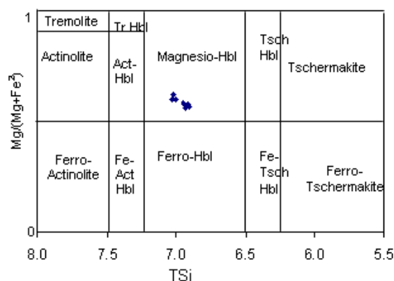
شکل ۵ نمودار نام‌گذاری آمفیبول‌ها [۷]، آمفیبول‌ها بیشتر در زیر رده‌ی مگنیو هورنبلند قرار می‌گیرند.
