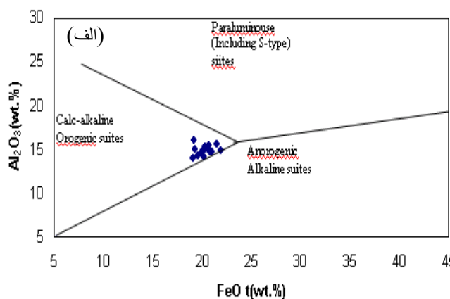
شکل ۹ الف و ب ترسیم اکسیدهای Al_2O_3 و FeO ، MgO بیوتیت‌های مورد بررسی در نمودارهای [۲۴].
