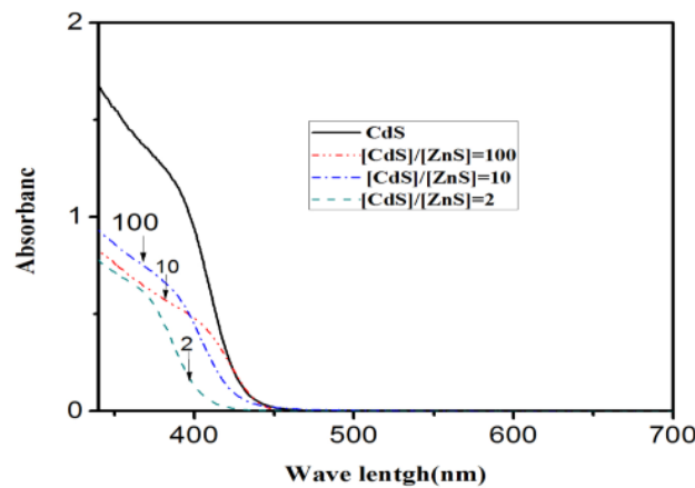
شکل ۲ طیف جذب نانوذرات CdS و [CdS]/[ZnS] = ۲, ۱۰, ۱۰۰
