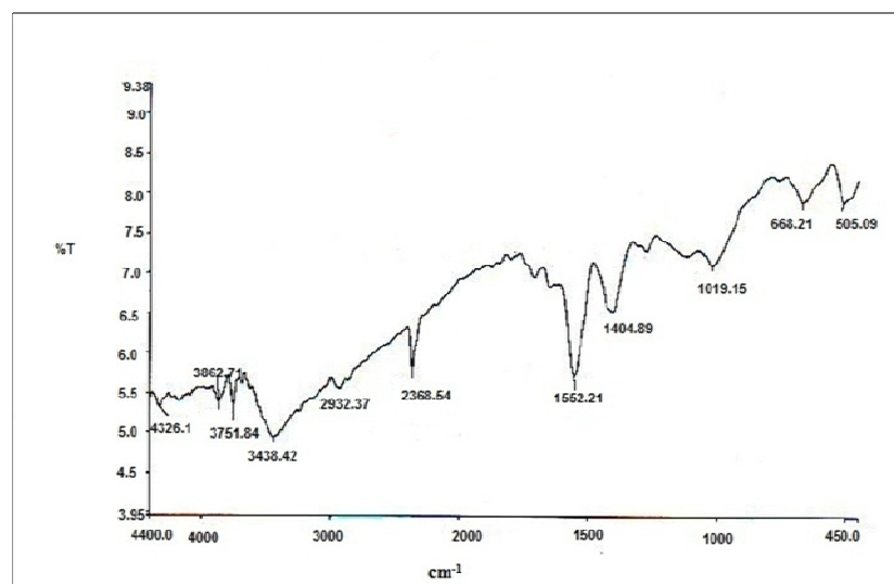
شکل ۷-ب طیف FTIR نانوذرات پوسته‌ی/هسته CdS/ZnS.
