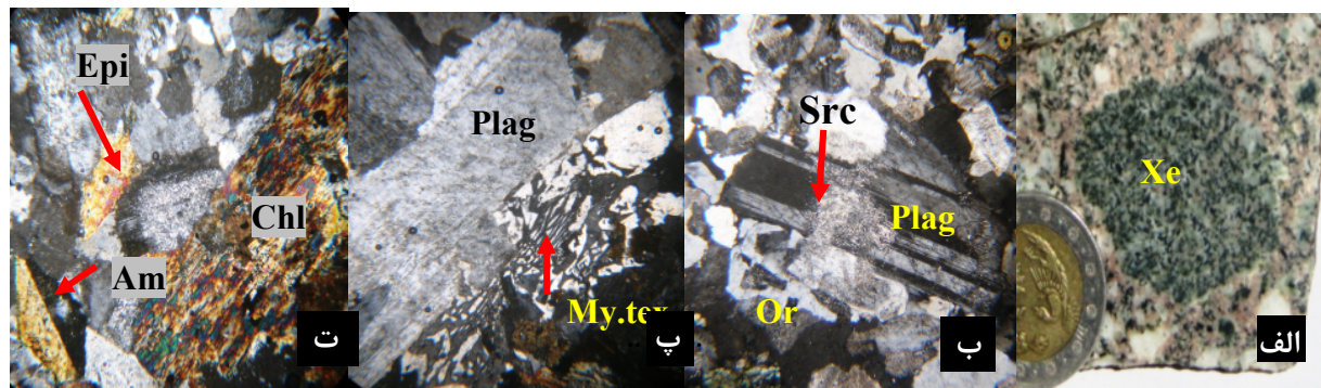
شکل ۵ الف- وجود برونیموم (Xe) دیوریتی در نمونه‌ی دستی گرانودیوریت. ب- بلور پلاژیوکلاز (Plag) که از مرکز به سرسیت (Src) و به صورت بخشی به ارتوکلاز (Or) تبدیل شده است. پ- بافت میرمیکیتی (my.tex) در گرانودیوریت (بزرگنمایی 4x، نورقطبیده). ت- آمفیبول‌های (Am) کاملاً دگرسان شده به کلریت (Chl) و اپیدوت (Epi) در گرانودیوریت (بزرگنمایی 4x، نورقطبیده).
