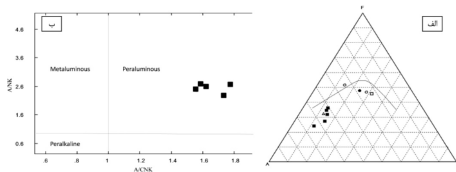
شکل ۶ الف) نمودار AFM سنگ‌های آذرین کانسار کهنک [۱۱]. ب) نمودار دسته‌بندی سنگ‌های آذرین بر اساس درصد اکسیدهای آلومینیوم، کلسیم، سدیم و پتاسیم [۱۲]. نمادها مشابه شکل ۴ هستند.
