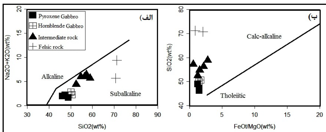
شکل ۴ الف) نمودار مجموع قلیایی نسبت به سیلیس [۸]. ب) نمودار (FeO^t/MgO) نسبت به SiO_2 ، برای جدایش گستره‌های آهکی-قلیایی و تولییتی [۹].
