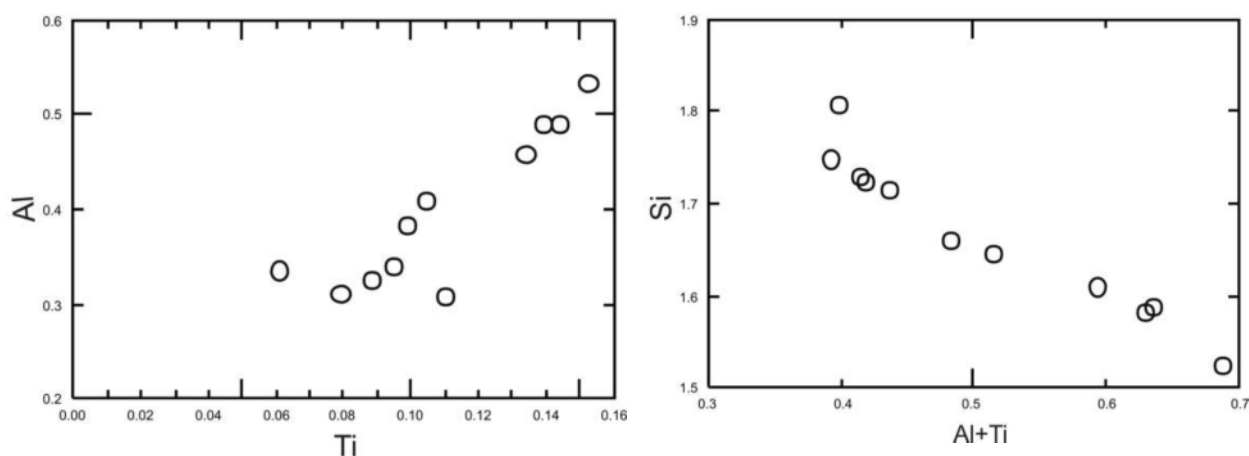
شکل ۷ روندهای مشاهده شده در کلینوپیروکسن‌ها که نشان‌دهنده تکامل شیمیایی کلینوپیروکسن‌ها به سمت غنی شدن از \text{Al} و \text{Ti} همراه با روند تبلور در این کانی‌هاست.
