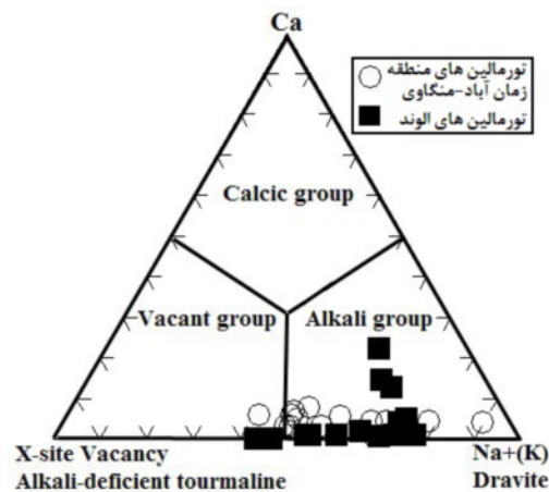
شکل ۴ نمودار مثلثی Ca-(X\text{-site vacancy})-Na+(K) [۱۴]، و موقعیت نمونه‌های مورد بررسی روی آن، X\text{-site vacancy}=1-(Ca+Na+K) .
