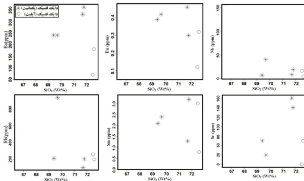
شکل ۷ نمودار عناصر فرعی در مقابل سیلیس [۱۸]، برای نمونه‌های دایک فلیسک (آپلیت و پگماتیت).
