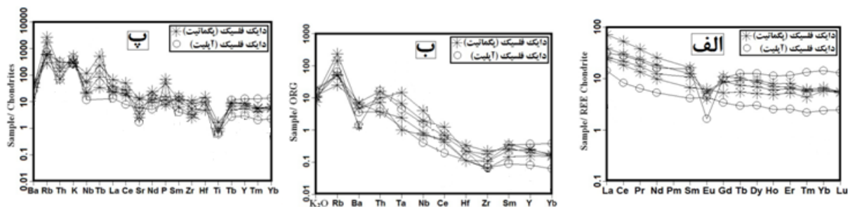
شکل ۸ نمودار عنکبوتی نمونه‌های دایک‌های فلیسک. الف) بهنجار شده با کندریت [۲۰]، ب) بهنجار شده با ORG [۲۱]، پ) نرمالیزه شده با کندریت [۲۲].
