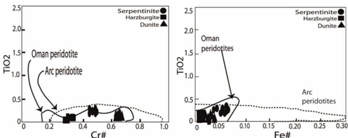
شکل ۴ (الف): نمودار \text{TiO}_2 در برابر عدد کروم اسپینل [۱۹]، (ب): نمودار \text{TiO}_2 در برابر عدد آهن Y_{\text{Fe}^{3+}} = [\text{Fe}^{3+} / (\text{Fe}^{3+} + \text{Cr} + \text{Al})] [۲۰، ۸]. نمونه‌های دونیت، هارزبورژیت و سرپانتینیت افیولیت شمال غرب پیرانشهر در موقعیت مشابه با موقعیت پریدوتیت‌های افیولیت عمان قرار گرفتند.
