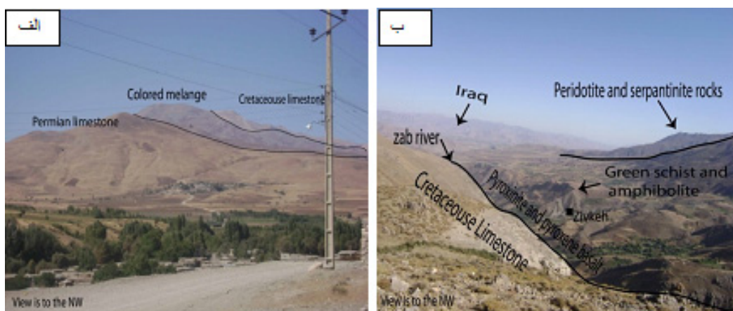
شکل ۲ (الف) آهک‌های پرمین، مجموعه‌ای در هم آمیخته افیولیت شمال غرب پیرانشهر، آهک‌های کرتاسه مجموعه افیولیتی را پوشانده است. (ب) موقعیت سنگ‌های مجموعه افیولیت شمال غرب پیرانشهر در نزدیکی مرز عراق.
