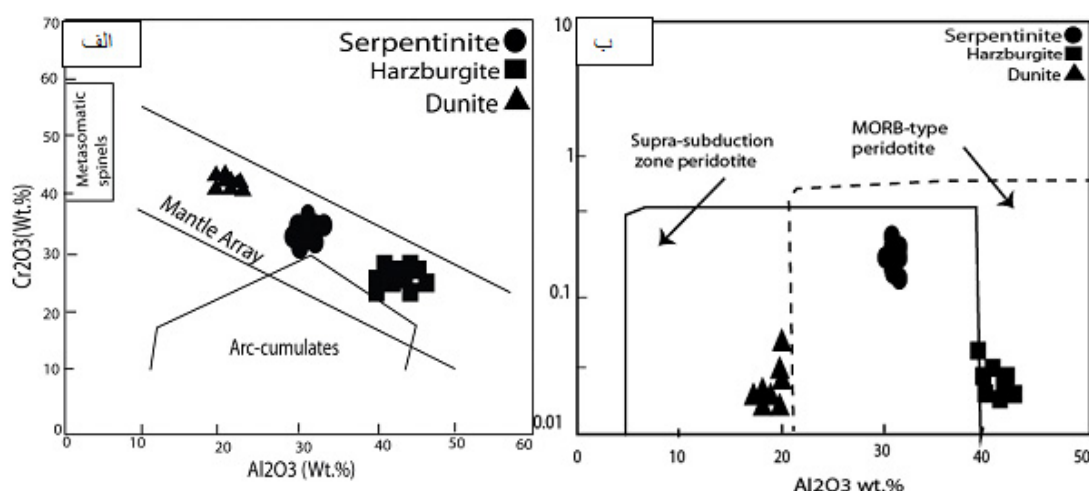
شکل ۵ (الف): نمودار درصد وزنی \text{Al}_2\text{O}_3 در برابر \text{Cr}_2\text{O}_3 اسپینل [۲۴]. نمونه‌های دونیت، هارزبورژیت و سرپانتینیت افیولیت شمال غرب پیرانشهر در محدوده‌ی الیومین - اسپینل شاخص گوشته (OSMA) قرار می‌گیرند. (ب): نمودار درصد وزنی \text{Al}_2\text{O}_3 در برابر \text{TiO}_2 اسپینل [۷]. دونیت در موقعیت پریدوتیت‌های ابرفرورانشی، هارزبورژیت در موقعیت پریدوتیت‌های پشته‌ی میان اقیانوسی، سرپانتینیت در همپوشانی محیط ابرفرورانشی و پشته میان اقیانوسی قرار گرفتند.
