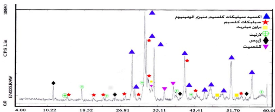
شکل ۱۱ بر پایه‌ی پراش پرتو ایکس (XRD)، سیمان نکهاء از اکسید سیلیکات کلسیم منیزیم آلومینیوم (اکسیدهایی که در اثر پخت ناقص مواد اولیه در کوره تولید می‌شوند) و سیلیکات کلسیم (تری کلسیم سیلیکات، دی کلسیم سیلیکات) تشکیل شده‌اند.
