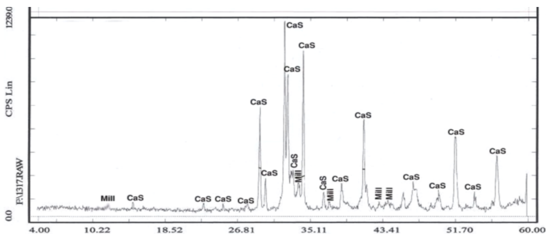
شکل ۱۰. پراش پرتو ایکس (XRD) کلینکر کارخانه سیمان نکاء. CaS = سیلیکات های کلسیم، Mill = براون میلیتریت.
