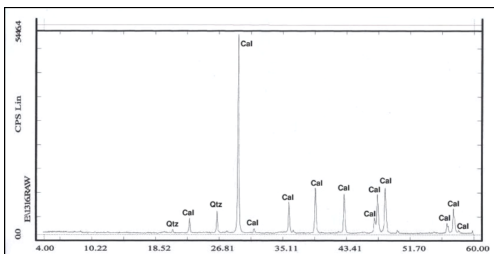
شکل ۱۲ نتایج پراش پرتو ایکس (XRD) غبار کوره سیمان نکهاء. Cal = کلسیت، Qtz = کوارتز.
