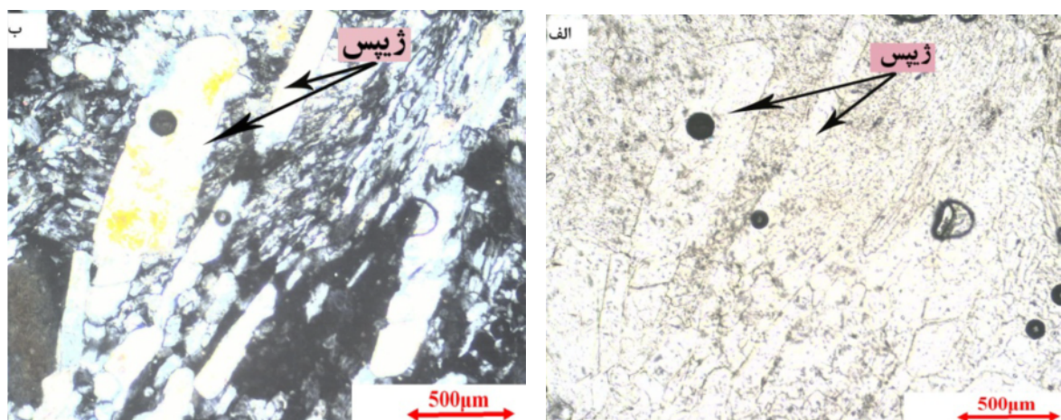
شکل ۴ مقطع میکروسکوپی سنگ گچ، الف، (PPL) و ب، (XPL). در آنالیزور رنگ‌های تداخلی شاخص ژئیس، خاکستری کم رنگ (نوع درجه یک) را می‌توان مشاهده کرد. ژئیس به دو صورت در مقطع میکروسکوپی سنگ گچ مشاهده شده است، به شکل شبکه‌ای از بلورهای نامنظم (گوشه سمت چپ تصویر) و به صورت رشته‌ای (مرکز تصویر).
