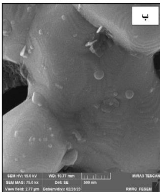
شکل ۶. تصاویر میکروسکوپ الکترونی روبشی گسیل میدانی نمونه آلاش داده شده با ۰/۵ کبالت الف) محدوده میکرومتر ب) محدوده نانومتر.
