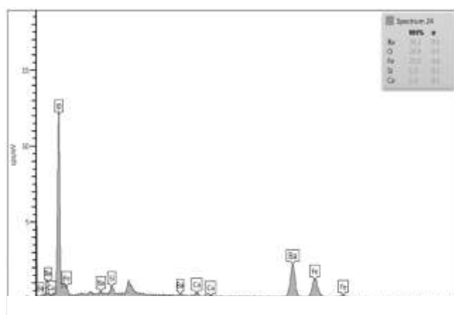
شکل ۵ تصاویر میکروسکوپ الکترونی روبشی (SEM) و طیف ED از کانی‌سازی باریت در منطقه آمین‌آباد.
