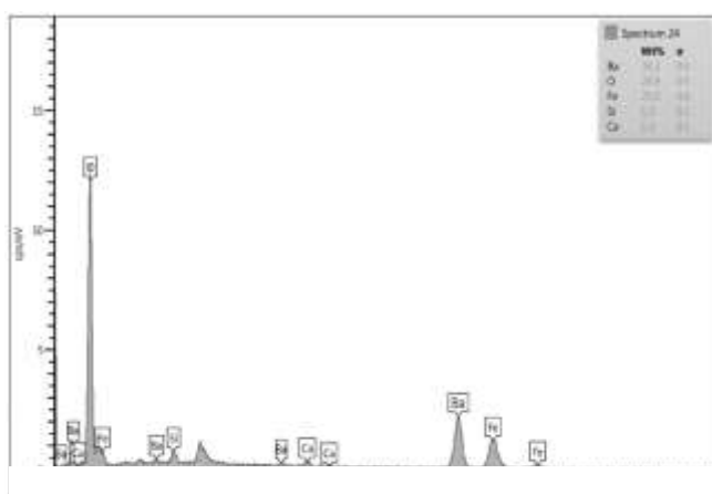
شکل ۵ تصویر میکروسکوپ الکترونی روبشی (SEM) و طیف EDX از کانی‌سازی باریت در منطقه آمین‌آباد.
