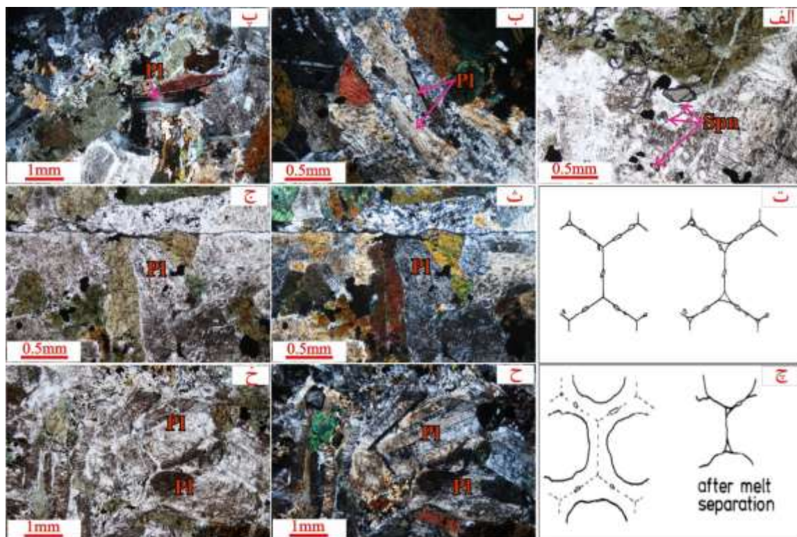
شکل ۶ الف) تیتانیت‌های با برجستگی بالا (در PPL)، ب) کانی پلاژیوکلاز قطعه شده نوع نوار برشی (در XPL)، پ) دگرشکلی خمیده در بلور پلاژیوکلاز، (در XPL)، ت) فازهای جانبی در مرزهای دانه (برگرفته از مرجع [۴۴])، ث) بلور پلاژیوکلاز با لبه مثلثی شکل (در XPL)، ج) بلور پلاژیوکلاز با لبه مثلثی شکل (در PPL)، چ) فازهای جانبی در مرزهای دانه (برگرفته از مرجع [۴۴])، ح) رگه آپلیتی و گردش‌گی در بلور پلاژیوکلاز با لبه گرد شده (در XPL)، خ) رگه آپلیتی و گردش‌گی در بلور پلاژیوکلاز با لبه گرد شده (در PPL)، اسفن و Pl: پلاژیوکلاز [۷].
