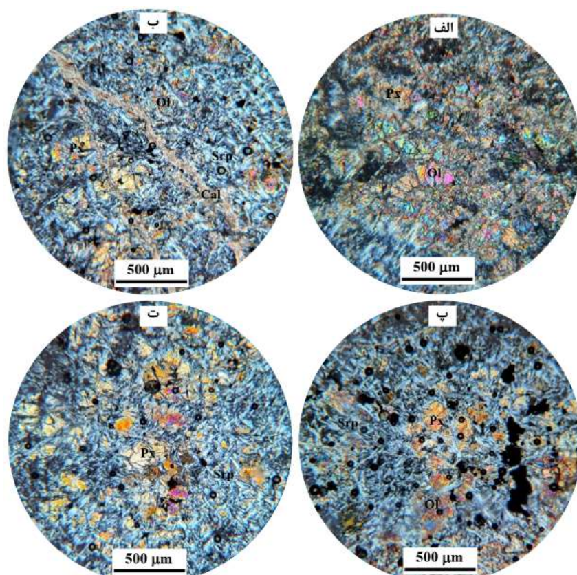
شکل ۳ تصاویر میکروسکوپی از واحدهای فرابازیک در منطقه قشلاق: الف) کانی‌های سنگ دونیت که شامل الیوین و به مقدار کم پیروکسن است، (ب) واحد دونیتی که به شدت سرپانتینیته شده و رگچه‌های کلسیت آنرا قطع کرده است، پ) کانی‌های تشکیل دهنده واحد هارژبورگیت که شامل پیروکسن و به مقدار کم الیوین است، ت) کانی‌های تشکیل دهنده واحد لرزولیت. Ol: الیوین، Px: پیروکسن، Cal: کلسیت، Srp: سرپانتین. [۱۸].
