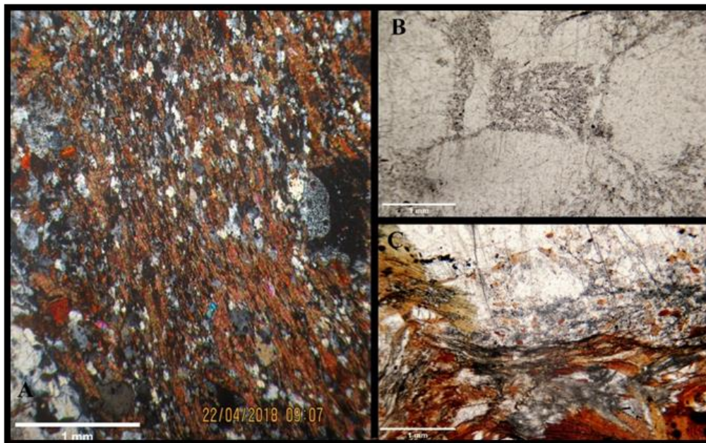
شکل ۵ الف) جهت‌یافتگی میکاشیست های منطقه قندآب در مقیاس میکروسکوپی همراه با جهت یافتگی ترجیحی ضعیف؛ (ب) حالت گرافیتی در بافت رشته‌ای فیبرولیت در دانه‌های آندالوزیت؛ (پ) بافت‌های پیچ و تاب خورده پیرامون شکفته بلورها همراه با رشته‌های فیبرولیت که می‌تواند نشانگر پیشروی دگرگونی باشد.
