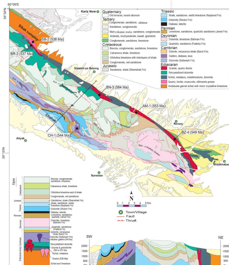
شکل ۱ - نمایی از منطقه مورد بررسی همراه با واحدهای زمین‌شناسی و ساختارهای منطقه و نیز برشی از مقاطع ساختاری موجود در مرکز عدسی - ساختاری و پهنه برشی فریمان - تربت جام نقشه ترکیبی لایه‌های زمین‌شناسی رقومی شده و نقشه زمین‌شناسی صد هزارم کارپزنو [۲].
