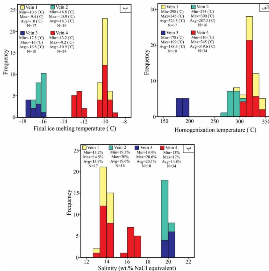
شکل ۶ نمودارهای ستونی مربوط به داماسنجی سیال‌های درگیر منطقه سماخون. الف) نمودار ستونی دمای همگن‌شدگی، ب) نمودار ستونی آخرین دمای ذوب یخ. پ) نمودار ستونی مقدار شوری.
