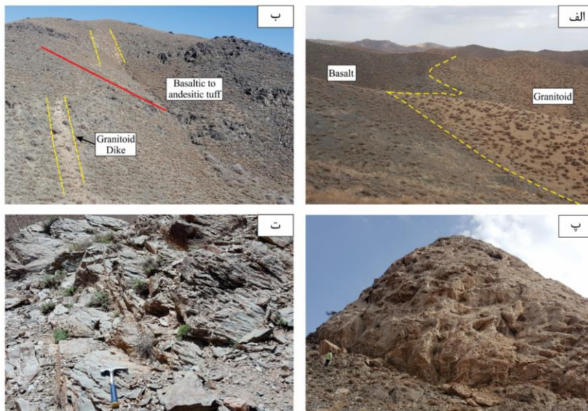
شکل ۳ رخنمون واحدهای سنگی منطقه سماخون؛ الف) نمایی از مرز بازالت با گرانیتوئیدها (دید به سمت جنوب شرق)، ب) رخنمون دایک گرانیتوئیدی درون توف بازالتی تا آندزیتی، پ) آهک (دید به سمت جنوب) و ت) ماسه سنگ.
